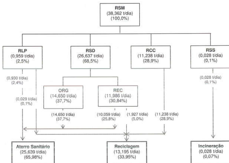
Figura 4: Fluxograma de resíduos sólidos do município de Pedreira.
